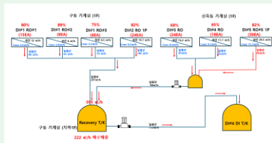
농축수 재이용 FLOW
